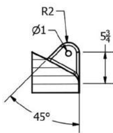
SECTION A-A SCALE 1:12
