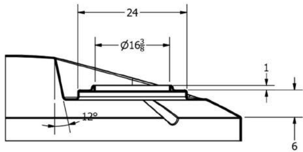
SECTION A-A SCALE 1:14
