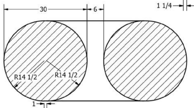
SECTION A-A SCALE 0.07 : 1
